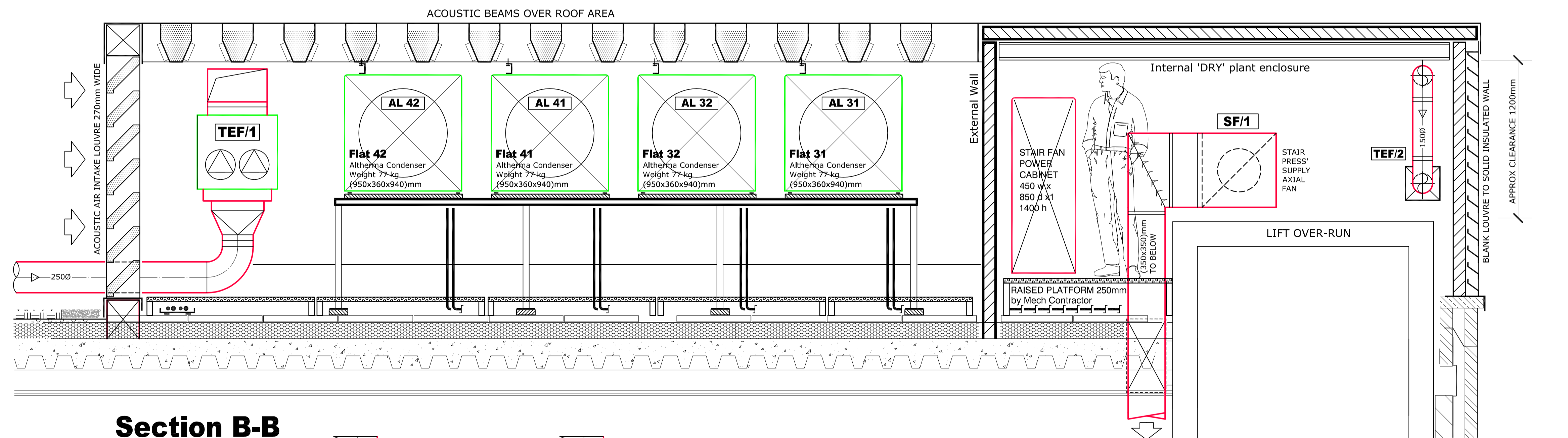
Section A-A
